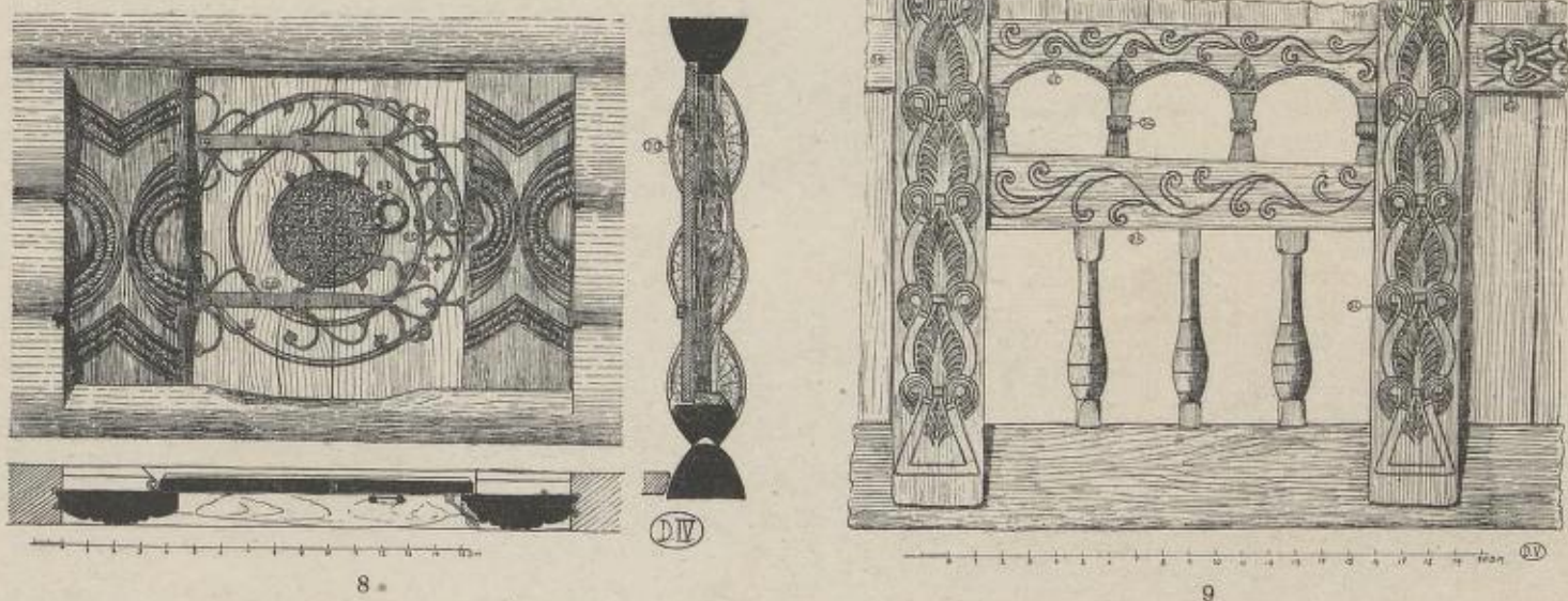
Detaljer frå Oselloftet. 1 glugg i svali (Pl. 34,1), st. 1:4. 2 detalj frå framsvali (sjå 9), st. 1:4. 3 dørringen (sjå 6 og 8), st. 1:2. 4 detalj av grind i tropi (Pl. 34, 1) st. 1:4. 5 detalj frå hyrnestolpane i svali (sjå 7), st. 1:4. 6 bursdøri. 7 hyrnestolpe. 8 loftsdøri. 9 gluggane i framsvali.
