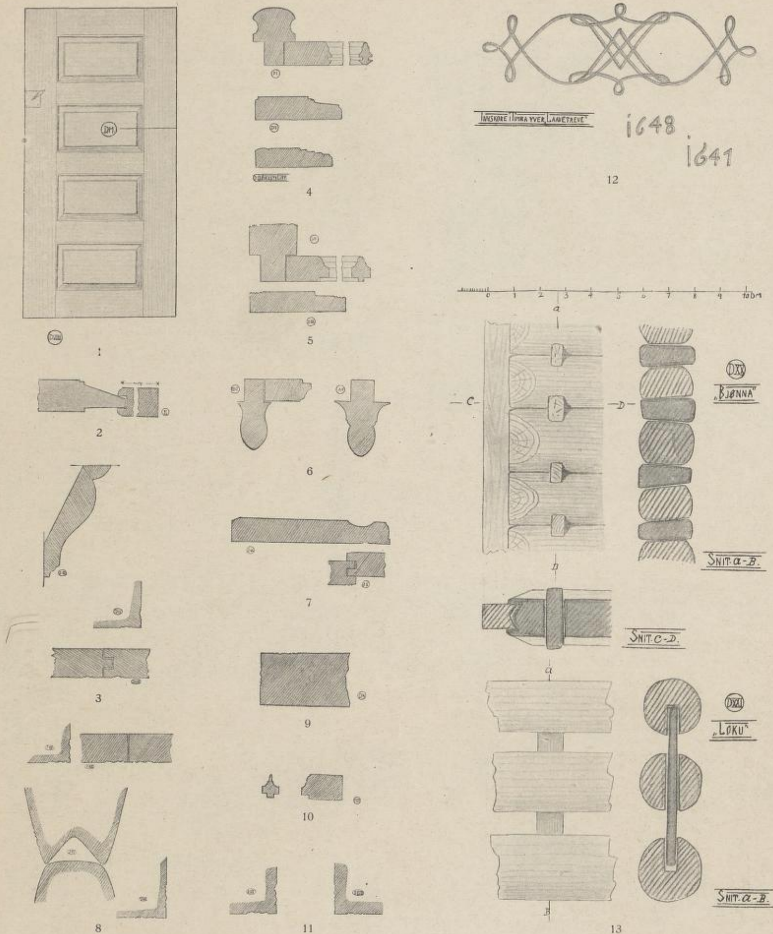
Brottveit, Valle. 1 og 2 kammerdøri på skjeldtile, st. 1:20, med detalj (Pl. 14, 5). 3-5 detaljer frå gl. og nyestog (Pl. 12, 5 og 13, 2). 6 og 7 detaljer frå skjeldtile (Pl. 14, 5). 8 og 9 detaljer frå loftet (Pl. 14, 1 og 3 og 18, 4). 10 detalj frå fjuset (Pl. 14, 4). 11 detalj frå låven (Pl. 15, 2). 12 og 13 detaljer frå løda (Pl. 16, 3 og 5). Alle detaljer, der det ikkje er påsett målestokk, er i kvart storleik.
