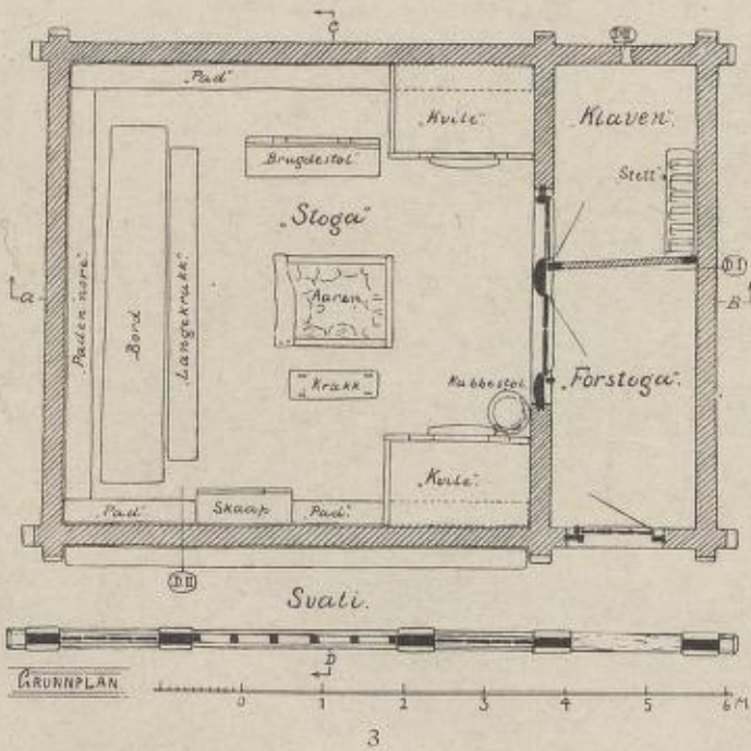
1—3 gamlestoga frå Aamli, Valle, no på Norsk Folkemuseum, 4—6 „setabu“ frå Bø-Hylledalen, Valle, no på Norsk Folkemuseum.
