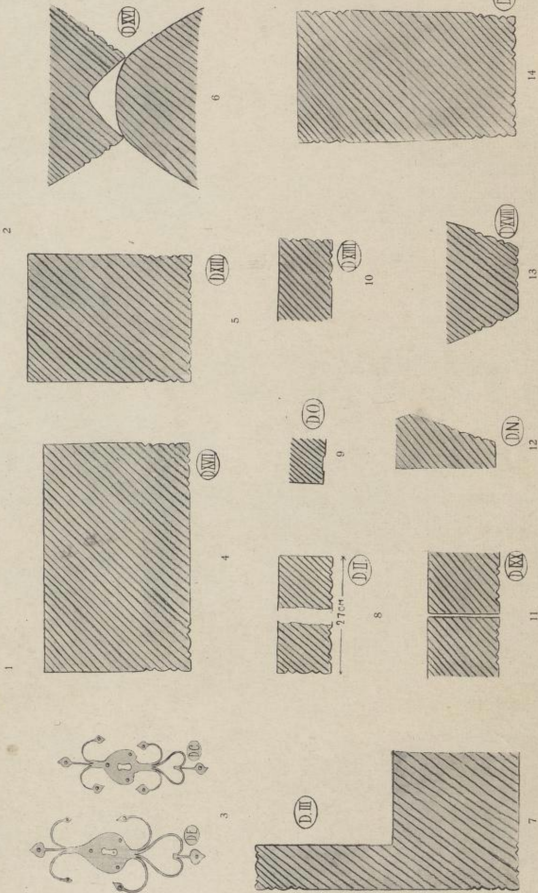
Detaljer frå Oseloftet. 1—3 hardjarn og lykleskrjå (Pl. 35, 6 og 8), st. 1: 10. 4, 5, 13 og 14 snitt av simsar, sperror, åsar og bjelkar (Pl. 34, 1 og 2), st. 1: 4. 6 og 9 snitt av timbra (Pl. 34, 1 og 2), st. 1: 2. 7 detalj av troppi (Pl. 34, 1 og 3), st. 1: 4. 8 snitt av stolpen under svali (Pl. 34, 4), st. 1: 4. 10 snitt av hyllone i loftet (Pl. 34, 1 og 2), st. 1: 4. 11 snitt av golvet i loftet (Pl. 34, 1), st. 1: 4. 12 snitt av stokken yver bursdøri (Pl. 35, 6), st. 1: 4.
