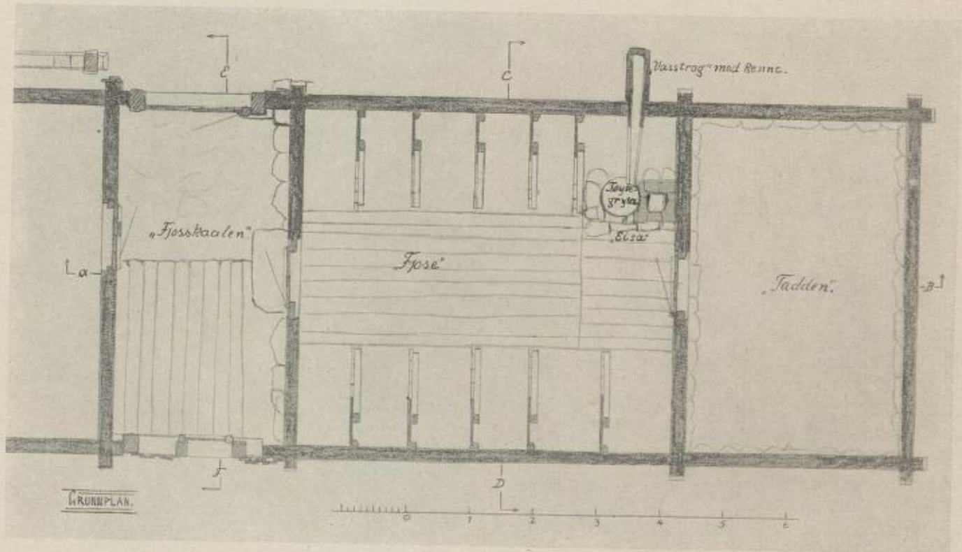
Fjos, Sygard Aakre, Valle.
