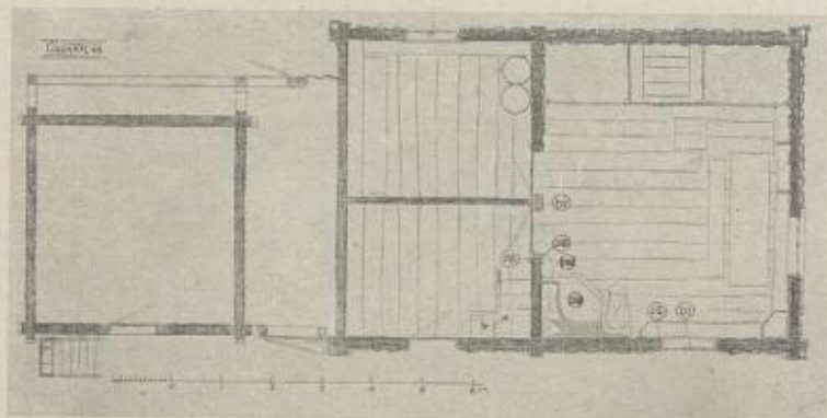
Grunnplan og detaljer fra nyestoga på Sygard Aakre, Valle. Detaljene i kvart storleik.
