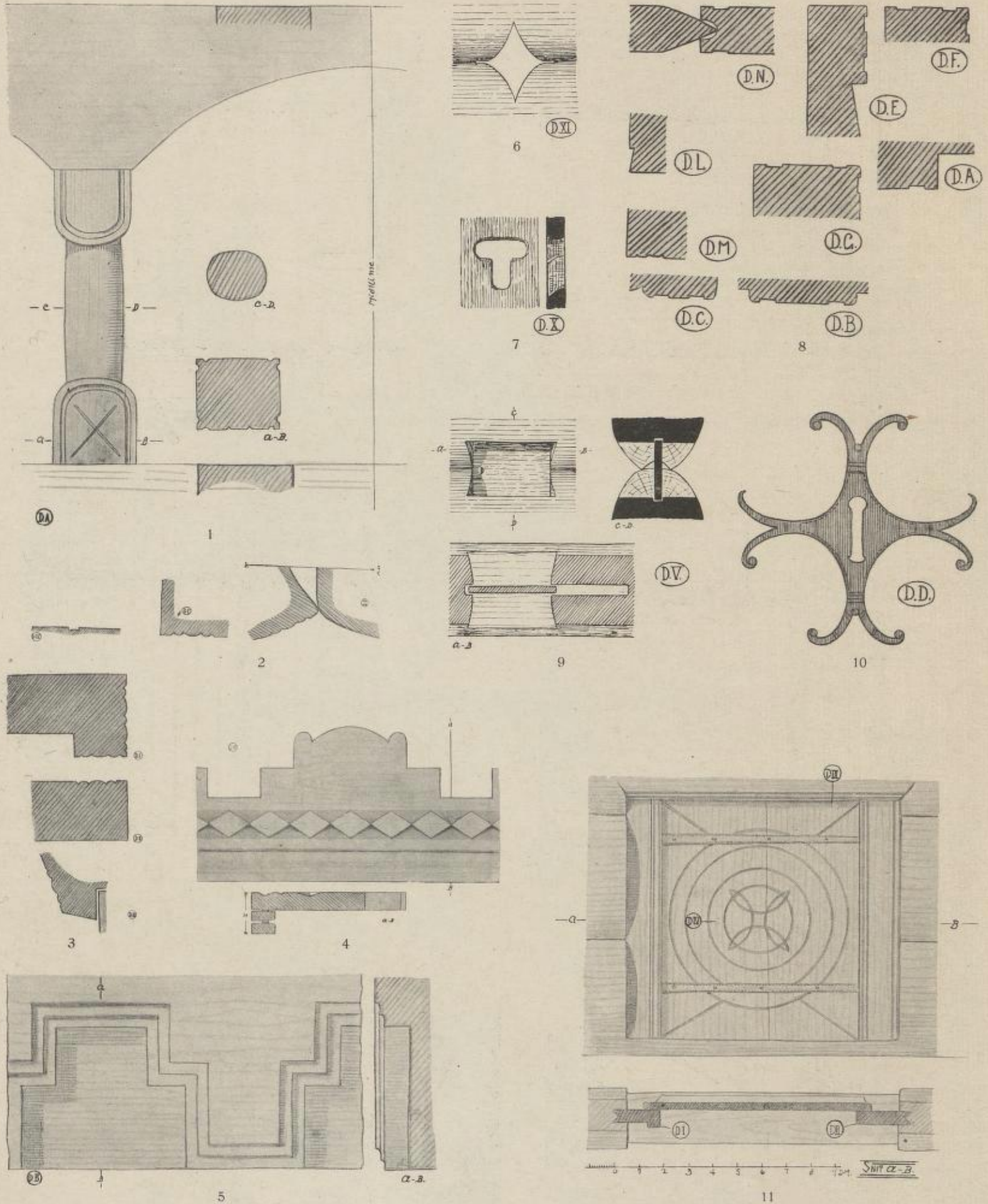
1—5 og 11 detaljer frå loftet på Dale, Valle. 1 detalj av loftsgluggane, st. 1:4. 2 detaljer av sperrone og timbra, st. 1:4. 3 detaljer av loftsdøri, st. 1:4. 4 hulle i loftet, st. 1:4. 5 detalj av svals villi til framsida, st. 1:4. 11 loftsdøri. 6—10 detaljer frå loftet på Haugen, Aaraksbø, Sandnes (Pl. 30 og 31). 6 og 9 gluggar i loftet, st. 1:10. 7 skjøteglugg (?) i svali, st. 1:10. 8 og 10 ymse detaljer frå svali, dørene og loftseingi, st. 1:4.
