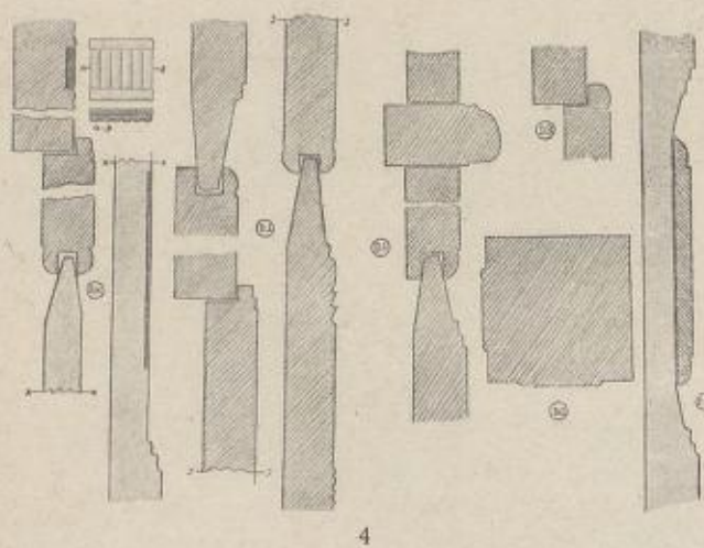
Brotteit, Valle. 1-5 „kvile“ og skåp med detaljer. 6-9 nyestogdøri med detaljer. Alle detaljer, der det ikkje er påsett målestokk, er i kvart storleik.
